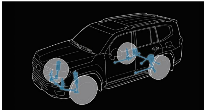
Новое поколение системы кинетической стабилизации подвески (E-KDSS)
